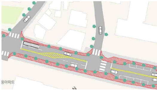
(a) 차도폭 좁힘 및 노상주차장 설치 도면
