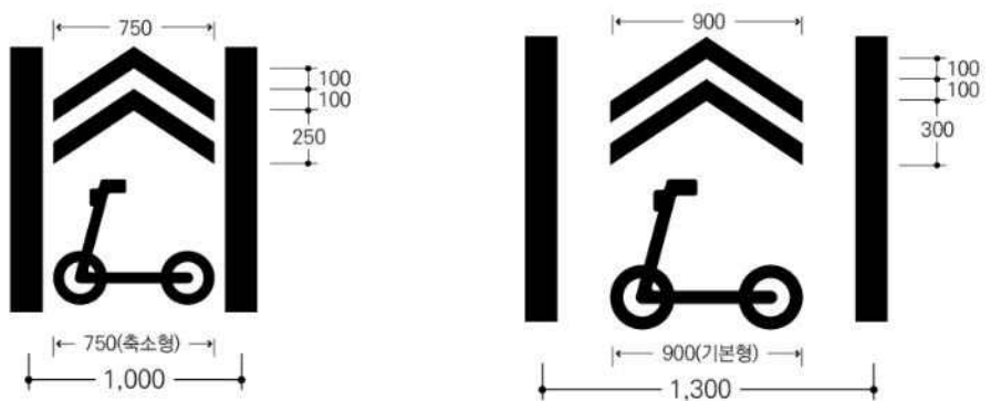
<그림 8-10> PM 우선도로 노면표시 예시
