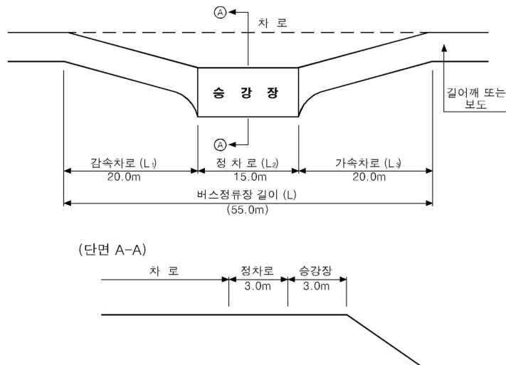
<그림 5-6> 간이 버스정류장(예시)
