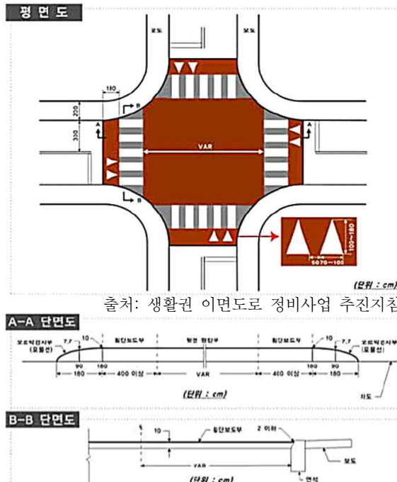
<그림 4-8> 고원식 교차로 설치 형상 및 제한
