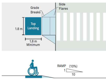
횡단보도 턱낮춤
