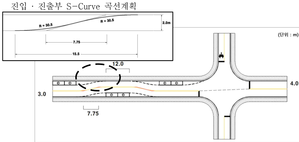
<그림 5-15> 지그재그 형태의 도로(교차로 진입부 주차면 설계)
