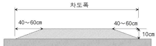
(b) 도로 횡단 방향
