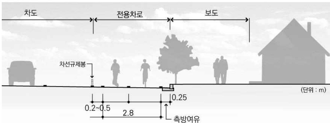
<그림 8-4> PM을 고려한 자전거 전용차로 횡단 예시
