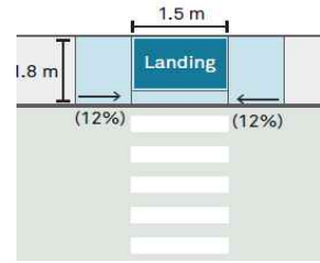
보도전체 턱낮춤
