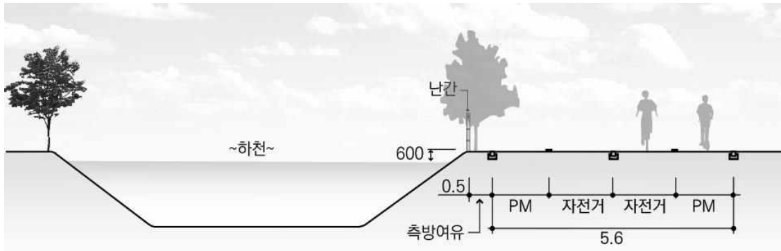
<그림 8-3> PM을 고려한 자전거 전용도로 횡단 예시(양방향)
