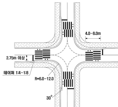
<그림 7-15> 교차로 폭 좁힘 제원
