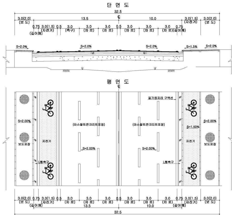
<그림 3-22> 설계속도 시속 40킬로미터일 때 자전거도로 설치 예시도(B=32.5m, 왕복 6차로)
